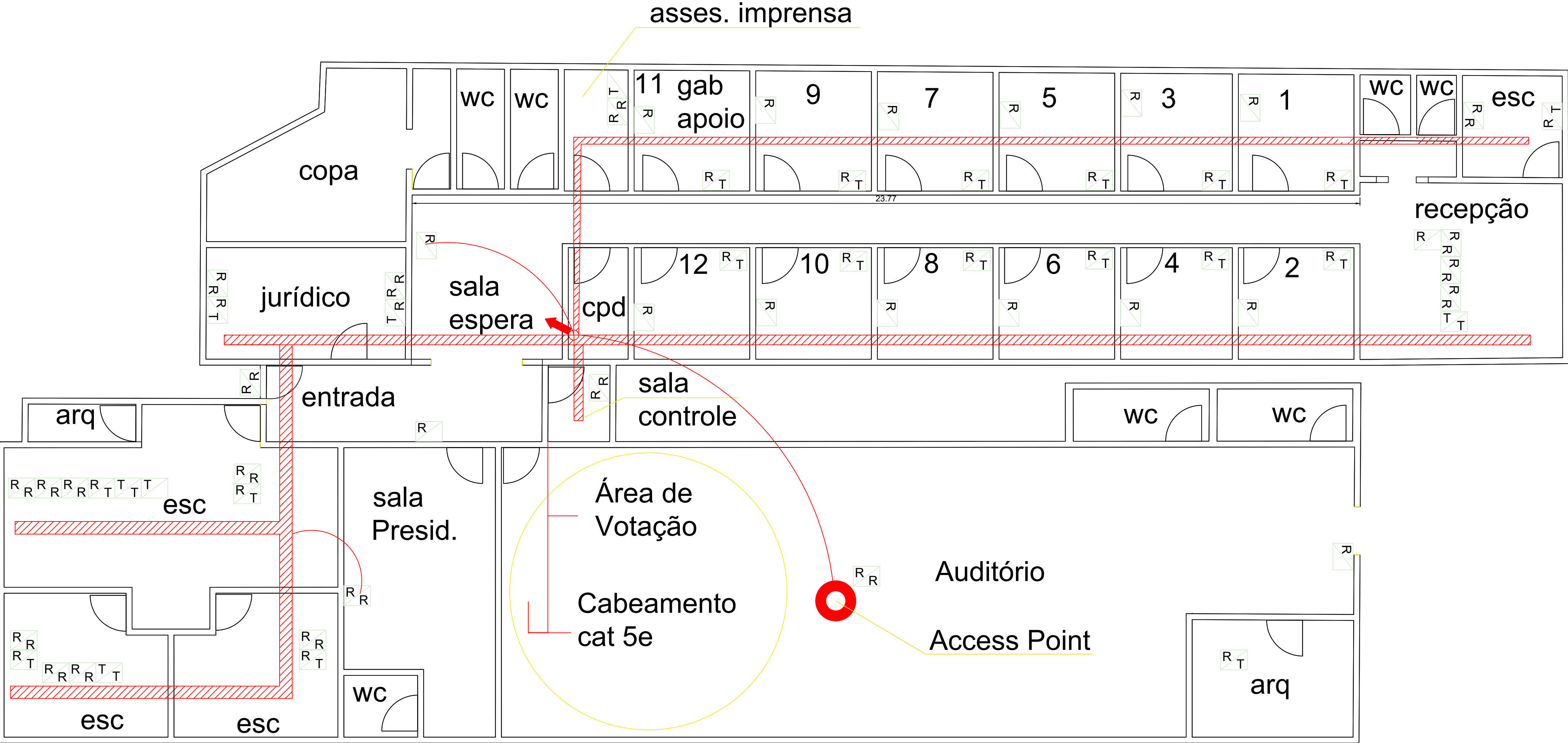
PLANTA BAIXA - CÂMARA MUNICIPAL
